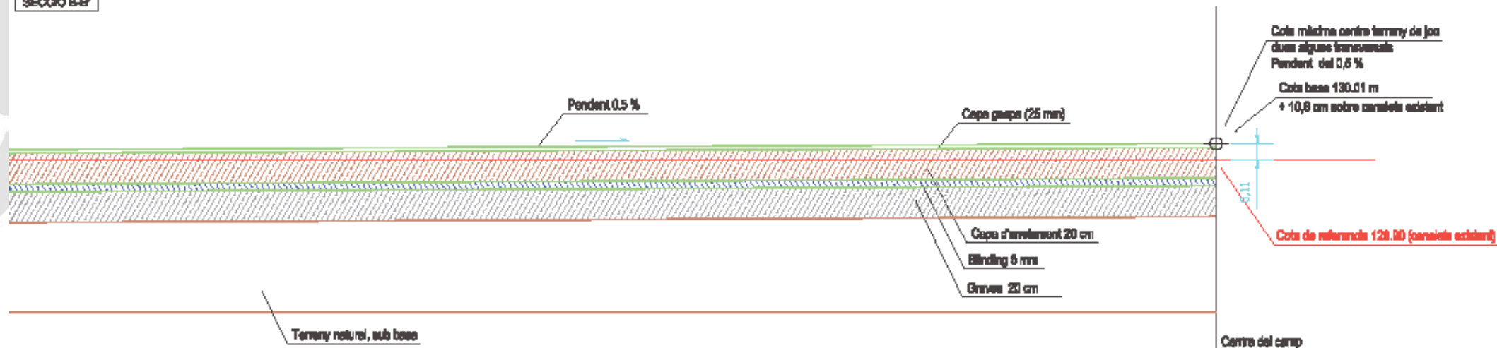
SECCIÓ B-B
