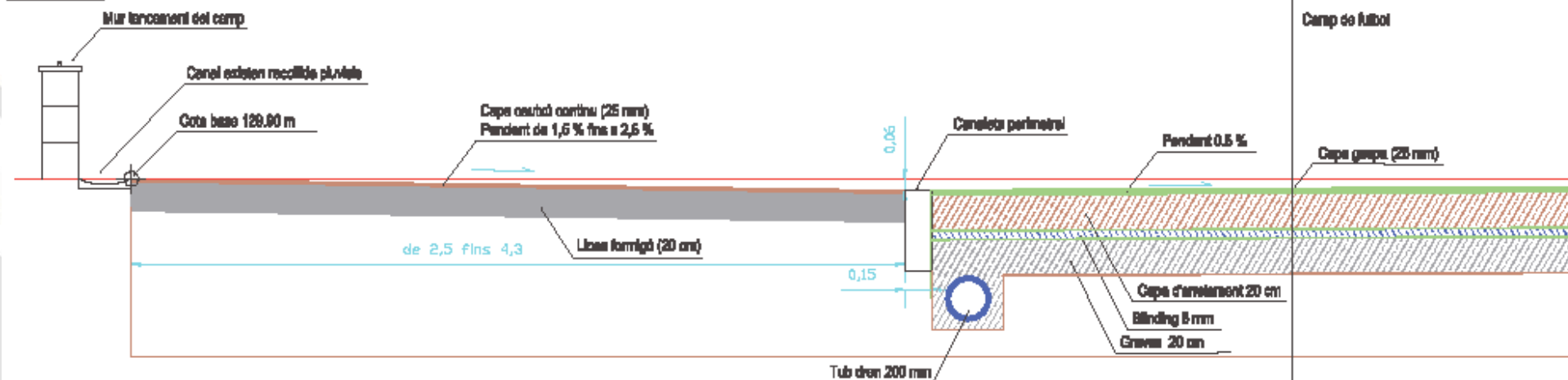
SECCIÓ A-A
